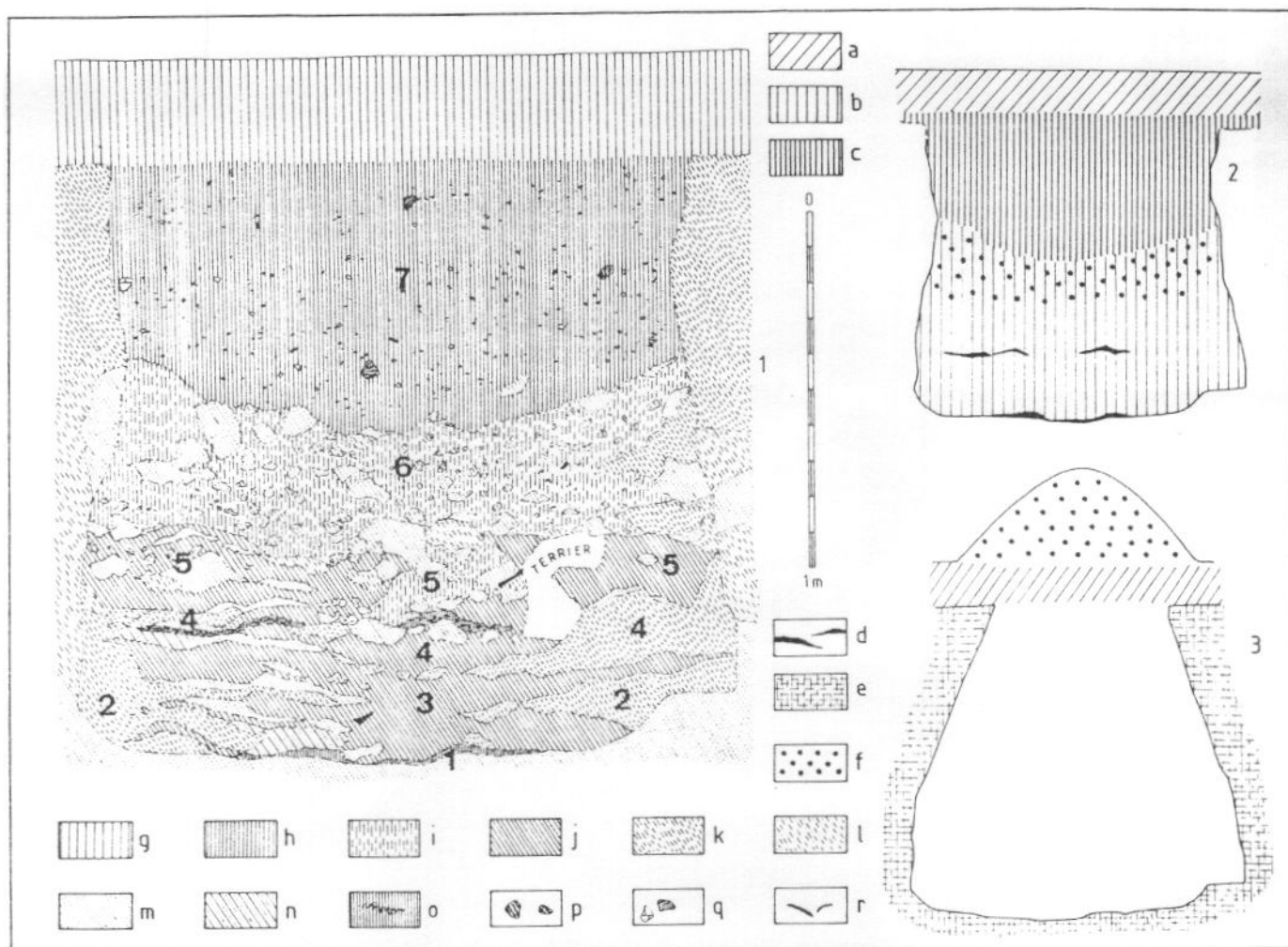
Fig. : silo n° 6 de Gidy : 1, relevé de la coupe ; 2, interprétation du remplissage ; 3, état supposé avant abandon (a et b - terre végétale, c - remblai artificiel, d et o - terre cendreuse et charbonneuse noire, e - sous-sol, f - cône supposé avoir protégé la fosse, g - remblai naturel, h - terre brune, i - mélange d'argile, de terre végétale, de calcaire jaune et de calcaire brun, j - terre argileuse brun-gris comportant du charbon de bois - k - argile rouge, l - calcaire brun altéré, m - calcaire jaune altéré, n - mélange de calcaire jaune et de terre argileuse, p - pierres étrangères au sous-sol, q - blocs calcaires brûlés ou non, r - tessons de poterie).
